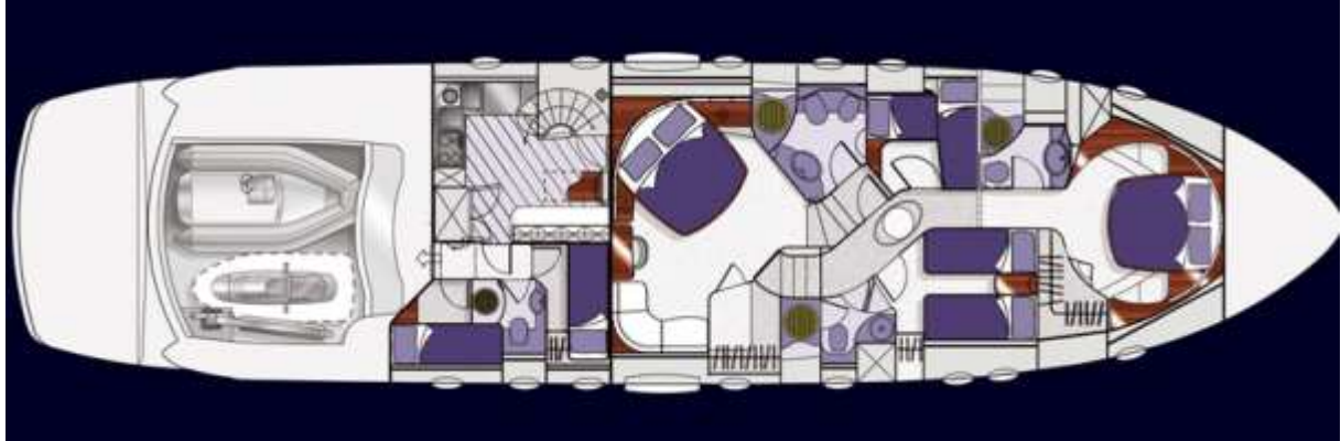
LOWER DECK LAYOUT PLAN DU PONT INFERIEUR
