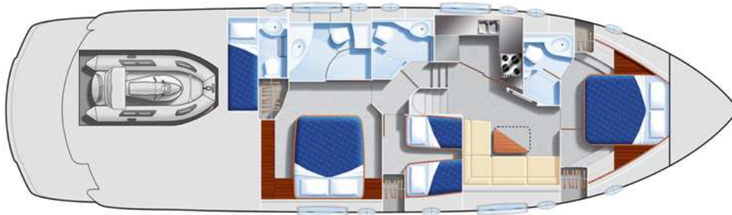
LOWER DECK LAYOUT PLAN DU PONT INFERIEUR
